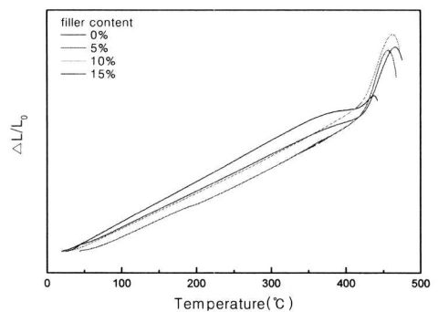
그림 4. 필러함량에 따른 전이점(°C), 연화점(°C), 열팽창계수( \times 10^{-7}/^{\circ}\text{C} ) 변화.
