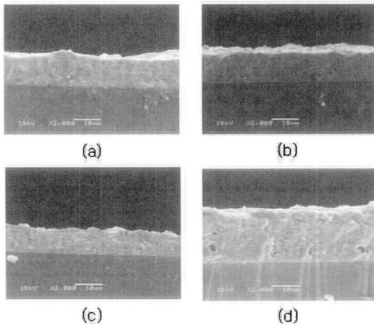
그림 2. 필러 함량의 15 %일 때, 열처리 온도 (a) 480 °C, (b) 500 °C, (c) 520 °C, (d) 540 °C 에서 20분간 열처리 시 횡단면의 SEM 사진.
