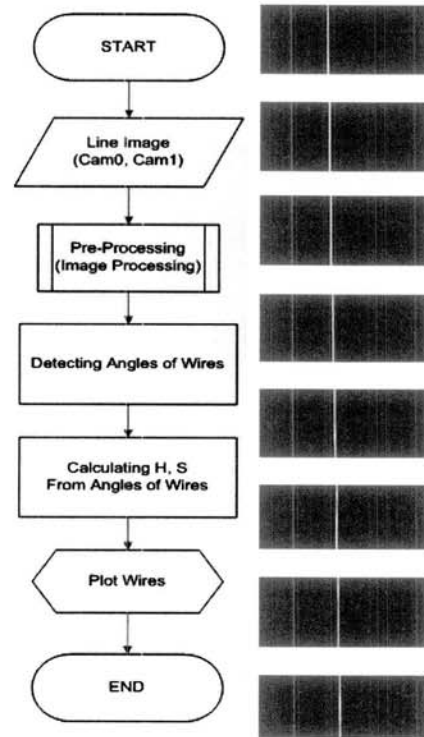
그림 5. 전차선의 검측 이미지 처리 과정 및 획득 이미지.
