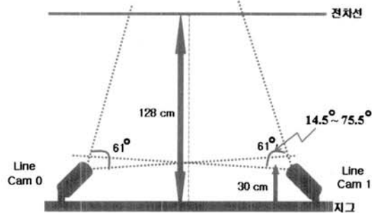
그림 3. 전차선 영상 획득 시스템 구조. Fig. 3. The overall structure of overhead contact wire monitoring system.
