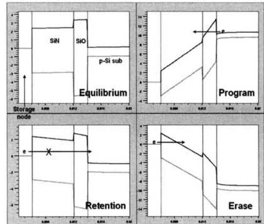
그림 3. 동작조건에 따른 에너지 밴드 구조 및 전자 터널링 상태.
