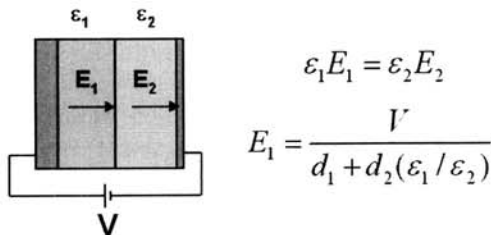
그림 2. 유전 상수가 다른 유전막을 적층시킨 경우의 전계분포.
