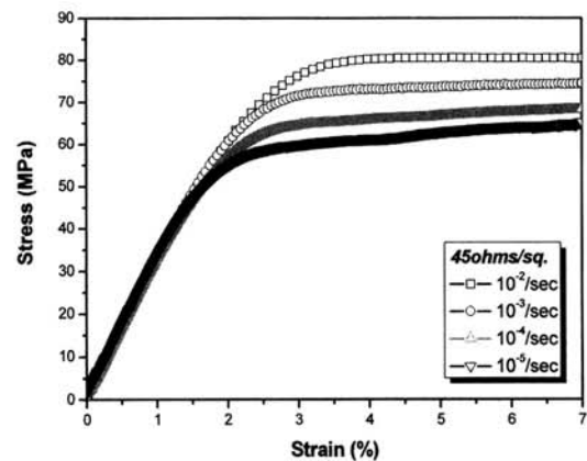
그림 2. 면저항 45 ohm/sq. ITO/PET 필름의 응력-변형률 그래프.
