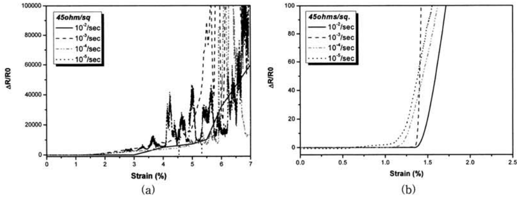
그림 3. (a) 변형률 속도에 따른 저항변화와 (b) 낮은 변형률에서의 저항변화. Fig. 3. \Delta R/R_o vs. strain curves at different strain rates (a) and the same at low strains (b).
