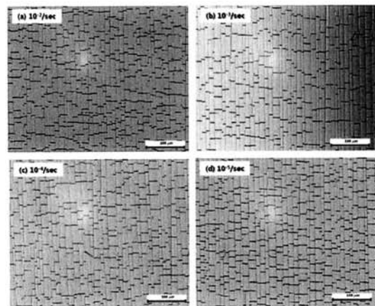
그림 9. 면저항 45 ohms/sq. ITO/PET필름의 변형률 속도에 따른 ITO층의 균열(7 % 변형률). Fig. 9. Cracks of ITO film with sheet resistance 45 ohms/sq. at different strain rate(7 % strain).
