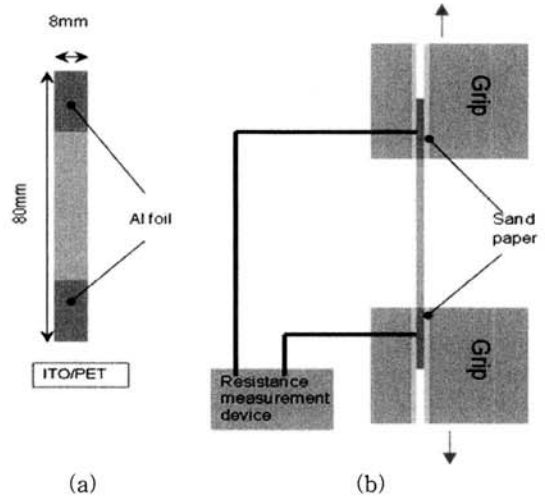
그림 1. (a)인장 시편과 (b)인장 시험 그림 및 장치 모식도.
