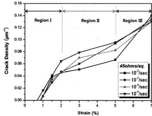
그림 4. 면저항 45 ohms/sq. ITO/PET 필름의 변형률 속도에 따른 균열 밀도. Fig. 4. Crack density of ITO/PET with the resistance of 45 ohms/sq. at various strain rates.
