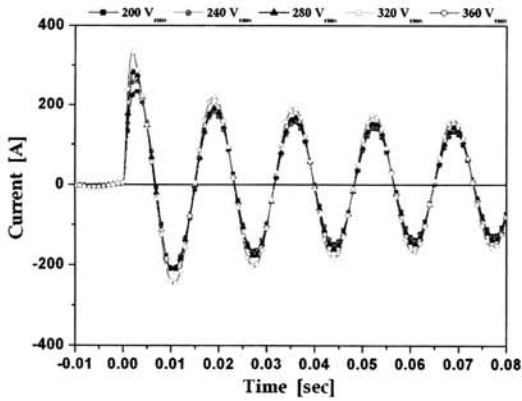
그림 7. 인가전압 변화에 따른 전류 특성 (R상 기준, 사고 각 45°, 1선 지락사고)
