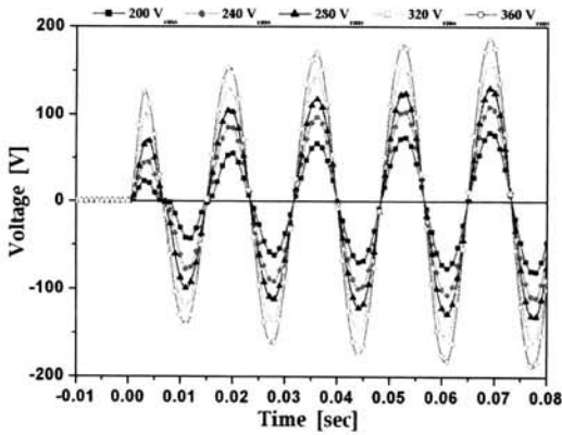
그림 8. 인가전압 변화에 따른 전압 특성 (R상 기준, 사고 각 45°, 1선 지락사고)
