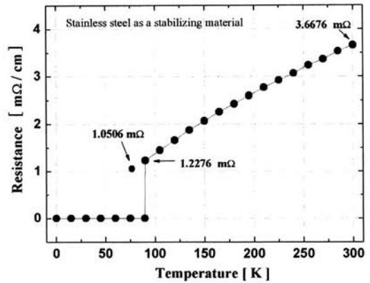
그림 2. YBCO coated conductor의 임계온도에 따른 저항 특성 곡선.
