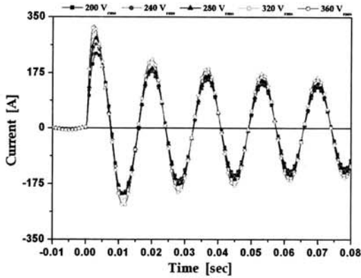
그림 4. 인가전압 변화에 따른 전류 특성 (R상 기준, 사고 각 0°, 1선 지락사고)
