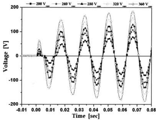
그림 11. 인가전압 변화에 따른 전압 특성 (R상 기준, 사고 각 90°, 1선 지락사고)
