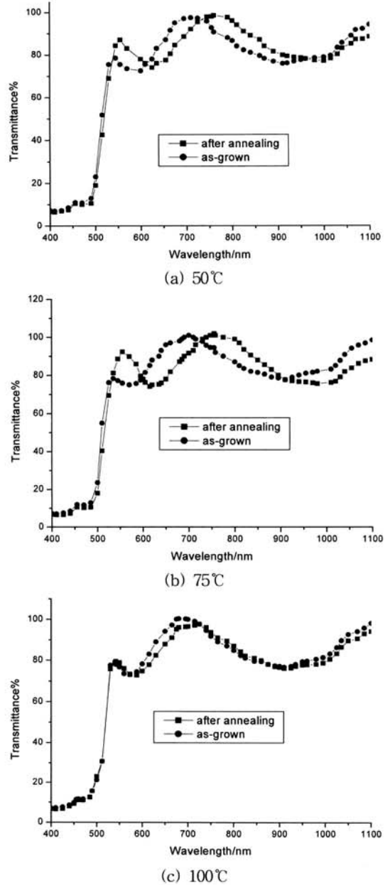
그림 5. CdS 막의 열처리 전·후의 광투과율. Fig. 5. Optical transmittance spectra of as-grown and after annealing CdS films deposited at different substrate temperatures.
