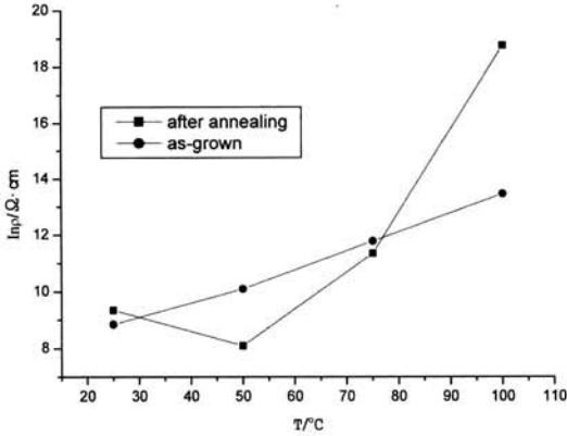
그림 8. 기판온도에 따른 저항율.
