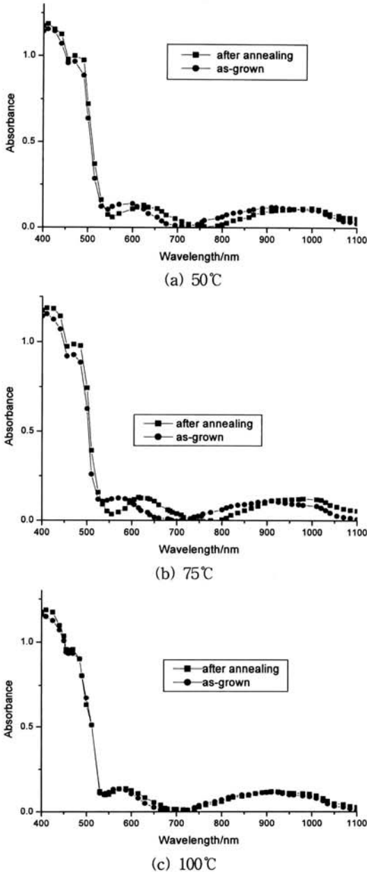
그림 6. CdS 막의 열처리 전·후의 흡수계수. Fig. 6. Absorbency spectra of as-grown and after annealing CdS films.
