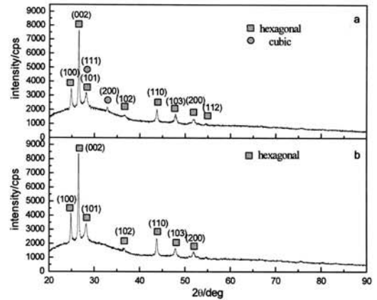
그림 2. 기판온도 50°C에서 증착된 CdS 막의 XRD 패턴 : (a) 열처리 전 (b) 열처리 후.
