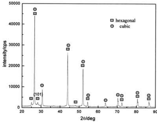
그림 1. CdS 분말의 XRD 패턴.
