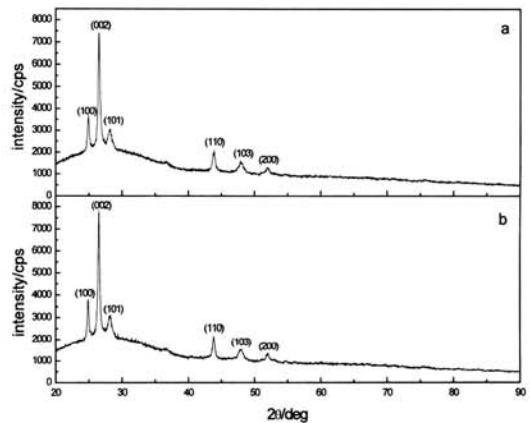
그림 3. 기판온도 100°C에서 증착된 CdS 막의 XRD 패턴 : (a) 열처리 전 (b) 열처리 후.
