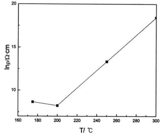
그림 7. 열처리 온도에 따른 저항율. Fig. 7. Dependence of resistivity on annealing temperatures.
