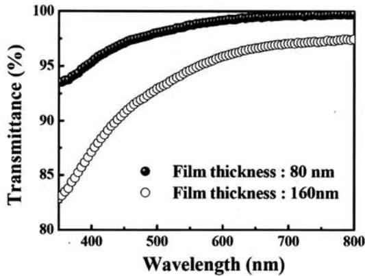
그림 4. 80 과 160 nm 두께의 Al 2 O 3 박막의 광 투과도.
