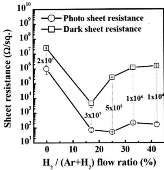
그림 2. 수소함량별 CdS 박막의 암실 및 노광 면 저항.
