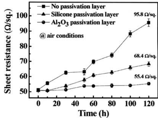
그림 5. CdS 박막위에 형성시킨 보호막층에 따른 시간별 노광 면저항의 변화.
