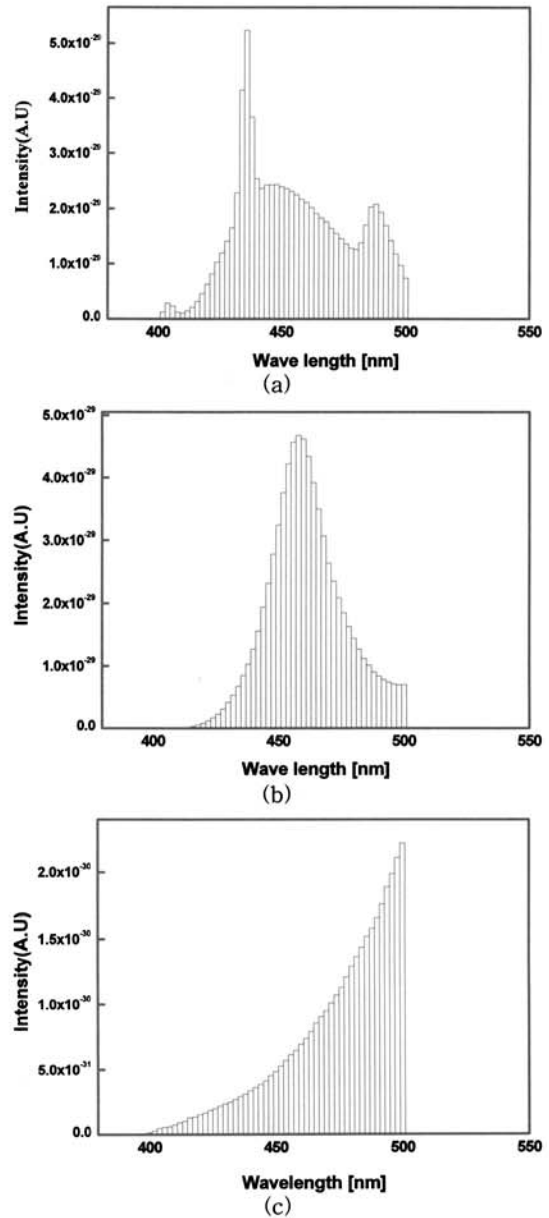
그림 3. 380~500 nm 파장의 범위에서 각 파장별 광자 에너지 및 파장별 스펙트럼의 intensity의 곱으로부터 계산된 광자 에너지 스펙트럼. (a) CCFL (b) white LED (c) halogen lamp Fig. 3. Photon energy spectral characteristics in a range of wavelength from 380 nm to 500 nm calculated from the multiplication of the photon energy and the spectral intensity at each wavelength (a) CCFL (b) white LED (c) halogen lamp.
