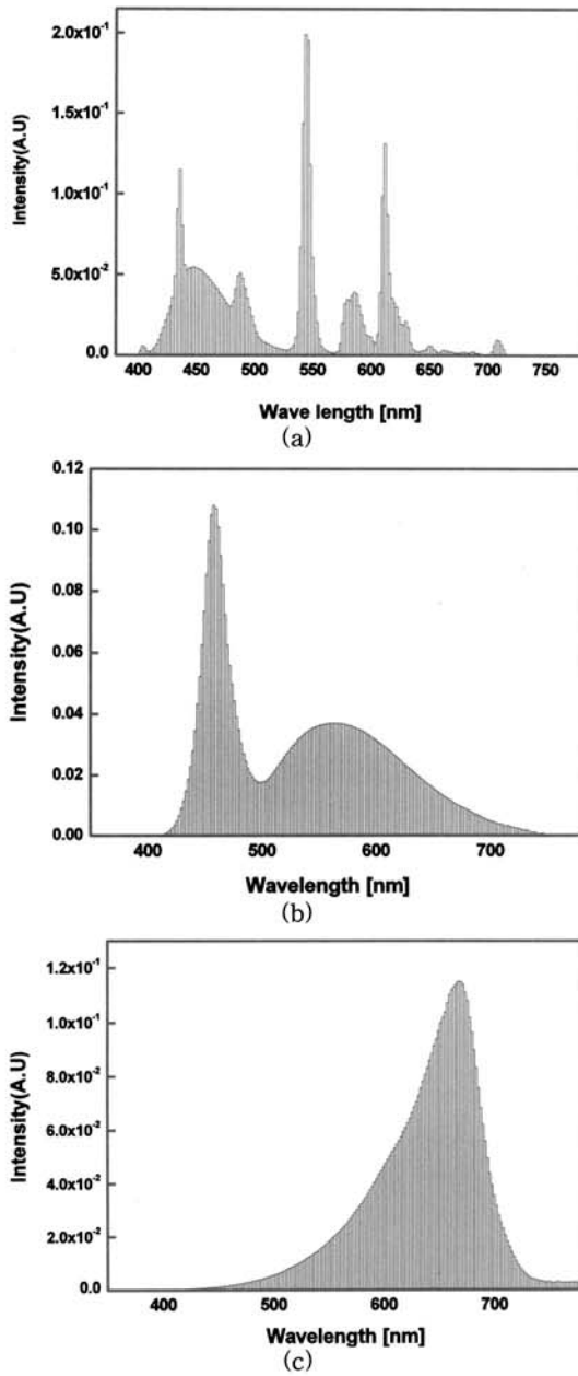
그림 2. 실험에 사용된 광원의 스펙트럼 특성. (a) CCFL (b) White LED (c) 할로겐 램프로 부터의 광자 에너지 스펙트럼 특성 Fig. 2. Spectral characteristics of the backlight used in the experiment, (a) CCFL (b) white LED (c) halogen lamp.
