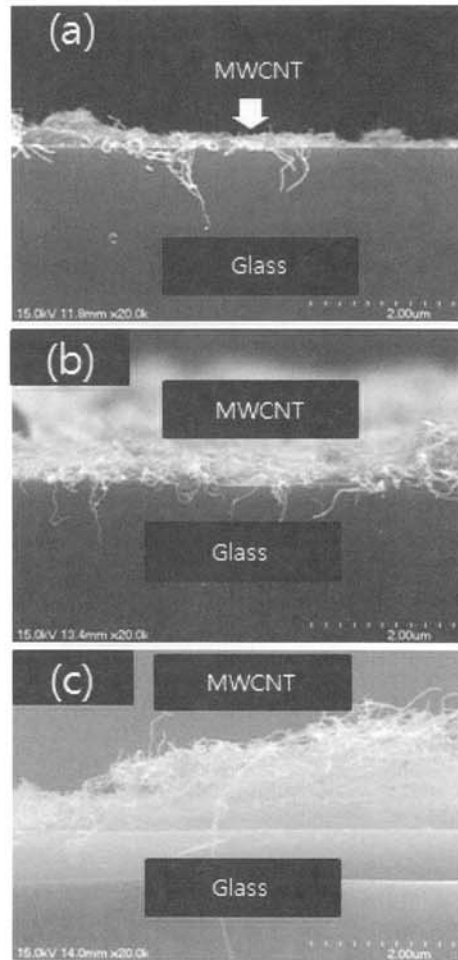
그림 4. MWCNT 스프레이 막의 SEM 단면.
