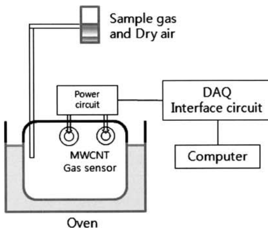
그림 2. 센싱계 측정장치도.
