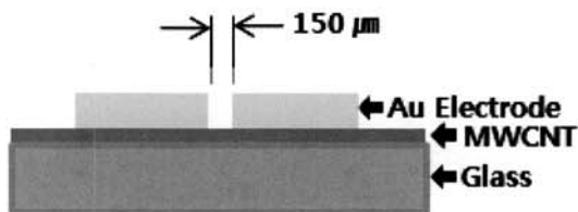
그림 1. 제작된 MWCNT 가스센서.
