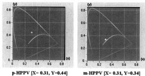
그림 8. p-HPPV와 m-HPPV EL 소자의 CIE 색좌표 그래프. Fig. 8. CIE color coordinates of EL devices based on p-HPPV and m-HPPV EL devices.
