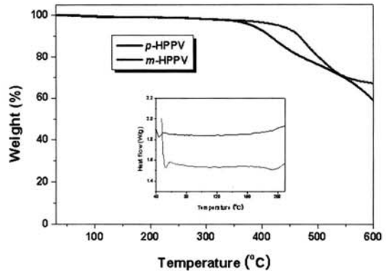
그림 9. p-HPPV와 m-HPPV의 TGA와 DSC 그래프. Fig. 9. TGA and DSC thermograph of p-HPPV and m-HPPV EL devices.
