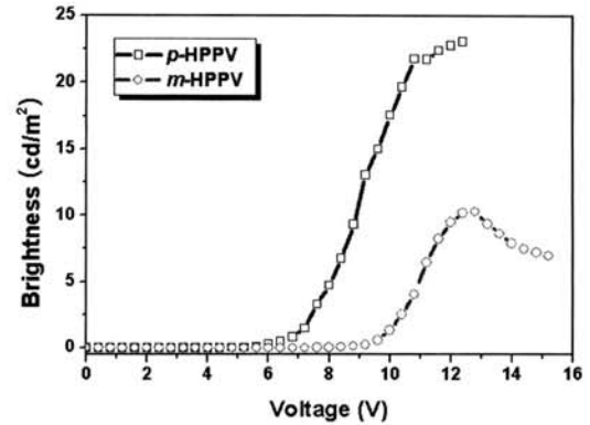
그림 6. p-HPPV와 m-HPPV EL 소자의 전압-휘도 그래프.
