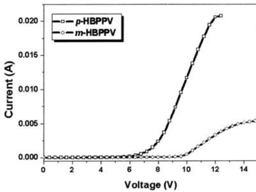
그림 5. p-HPPV와 m-HPPV EL 소자의 전압-전류 그래프.
