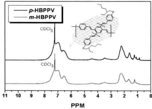
그림 2. p-HBPPV와 m-HBPPV의 1 H-NMR 스펙트럼. Fig. 2. 1 H-NMR spectra of p-HBPPV and m-HBPPV.
