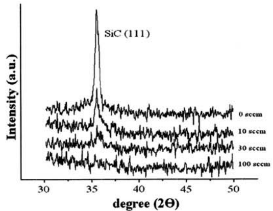
그림 2. N 2 in-situ 도핑량에 따라 성장된 다결정 3C-SiC 박막의 XRD 스펙트라.
