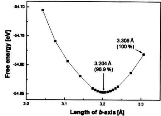
그림 1. Tetragonal-NiSi 구조에서 b 축의 길이 변화에 따른 에너지 변화.
