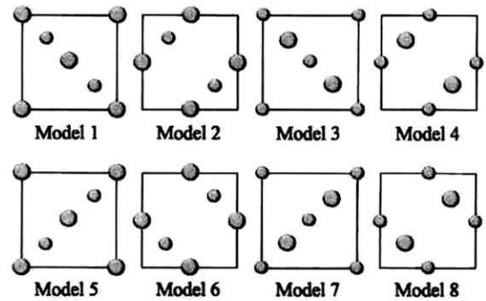
그림 2. 8개의 Si 표면 원자 배열. 원의 크기는 b 축의 좌표 변화를 의미한다.
