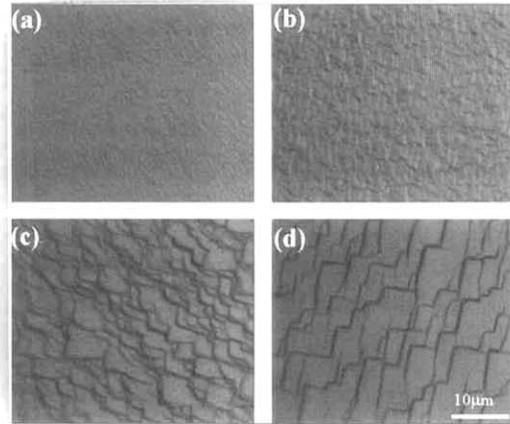
그림 3. 온도에 따라 (001)면에서 4° 기울어진 GaAs기판에 성장된 열전박막의 형상. (a) 300 °C (b) 380 °C (c) 400 °C (d) 450 °C Fig. 3. Surface morphologies of Bi-Sb-Te alloy layers on <001>GaAs substrates tilted 4° toward <010>grown at (a) 300 °C, (b) 380 °C, (c) 400 °C, and (d) 450 °C.
