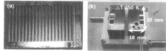
그림 5. 열전소자 및 측정치구.
