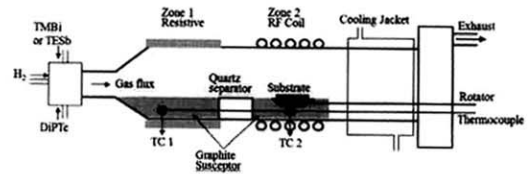
그림 1. MOCVD 반응관 구조.
