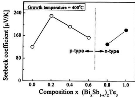
그림 4. (Bi_xSb_{1-x})_2Te_3 박막의 조성에 따른 상에서의 열전상수(Seebeck Coefficient).
