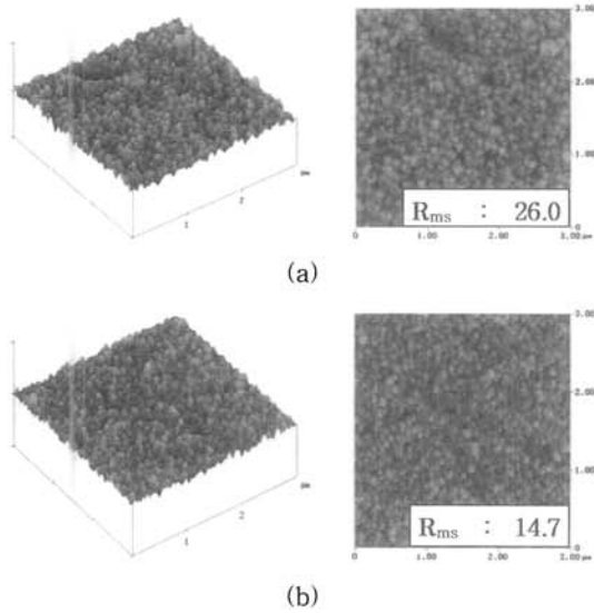
그림 4. ZnS/CaF 2 /ZnS/Cu 다층박막에서 CaF 2 광학두께 변화에 따라 제조된 다층막의 표면 AFM 이미지 : (a) 0.25 λ and (b) 0.5 λ. Fig. 4. AFM images in the ZnS/CaF 2 /ZnS/Cu multi-layered film depending on optical thickness of CaF 2 : (a) 0.25 λ and (b) 0.5 λ.
