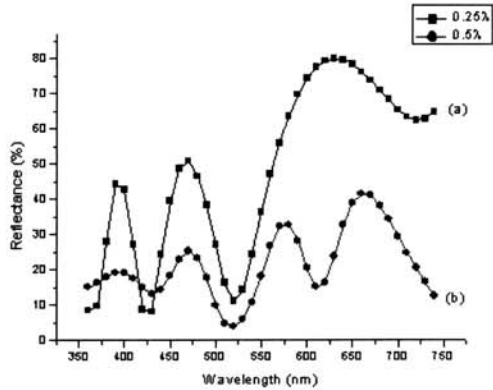
그림 6. CaF 2 광학두께 변화에 따라 제조된 ZnS/CaF 2 /ZnS/Cu 다층 박막의 광도계로 측정 한 반사율 변화 : (a) 0.25 λ and (b) 0.5 λ.
