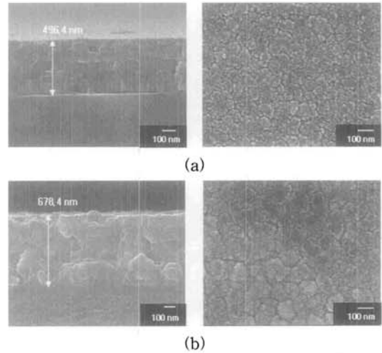
그림 3. ZnS/CaF 2 /ZnS/Cu 다층박막에서 CaF 2 광학두께 변화에 따라 제조된 다층막의 단면 SEM 사진 : (a) 0.25 λ and (b) 0.5 λ.
