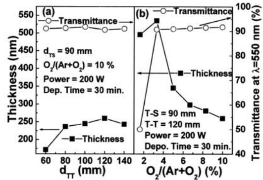
그림 4. (a) O 2 /(Ar+O 2 )=10 %인 조건에서 d TT 의 함수와 (b) d TT =120 mm인 조건에서 O 2 /(Ar+O 2 ) 산소 분압비의 함수에 따라 증착된 SiO x 박막의 두께 및 550 nm의 파장에서 측정된 광학적 투과율. Fig. 4. Thickness and optical transmittance (at λ=550 nm) of SiO x films deposited as a function of (a) parameters of d TT under O 2 /(Ar+O 2 )=10 % condition and (b) O 2 /(Ar+O 2 ) oxygen pressure under d TT =120 mm condition.
