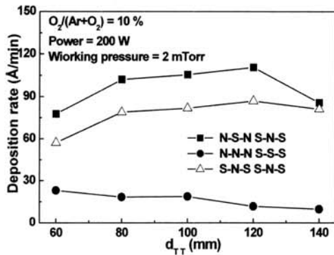
그림 3. 다양한 캐소드 자석 배열에 따라 제작된 SiO x 박막에서 d TT 의 함수에 따른 증착율. Fig. 3. Deposition rate as a function of d TT for SiO x films prepared under different cathode magnet arrangements.
