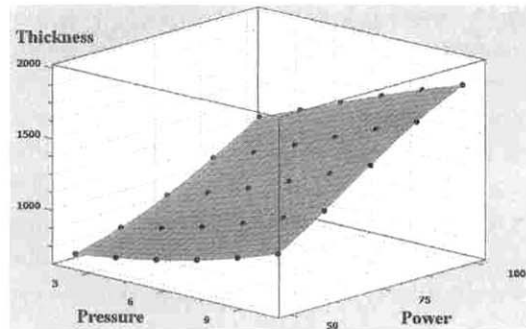
그림 1. DC파워와 챔버 압력에 따른 증착두께의 영향.
