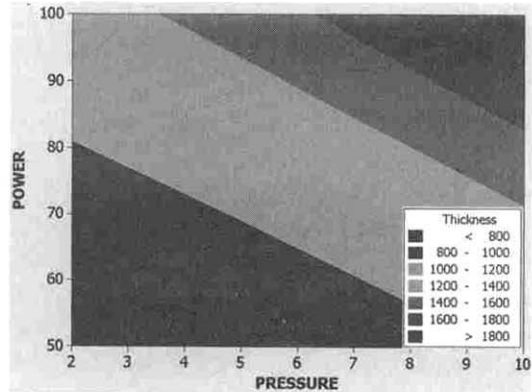
그림 2. DC파워와 챔버 압력에 따른 증착두께의 영향 등고선.
