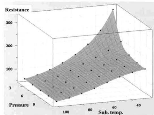
그림 3. 챔버 압력과 기판온도에 따른 박막 면저항의 영향.
