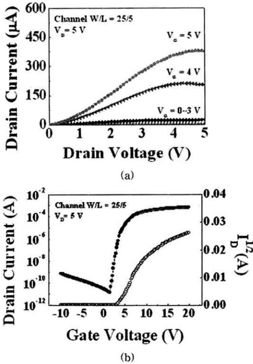
그림 3. 제작된 a-IGZO TFT (channel W/L = 25/5 μm)의 전기적 특성 (a) 출력 특성 (b) 전달 특성. Fig. 3. Electrical characteristics of the a-IGZO TFT (channel W/L = 25 μm/5 μm) (a) Output characteristics (b) Transfer characteristics.
