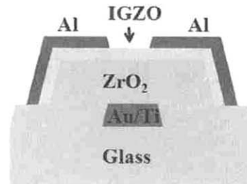
그림 1. a-IGZO TFT 단면도.
