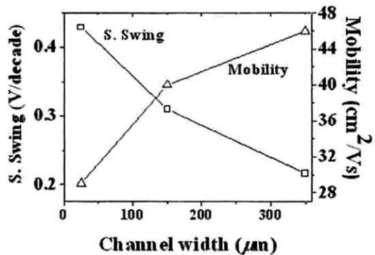
그림 5. 제작된 a-IGZO TFT의 채널 W/L에 따른 Subthreshold Swing값과 이동도 특성. Fig. 5. The subthreshold swing and field-effect mobility of a-IGZO TFT.
