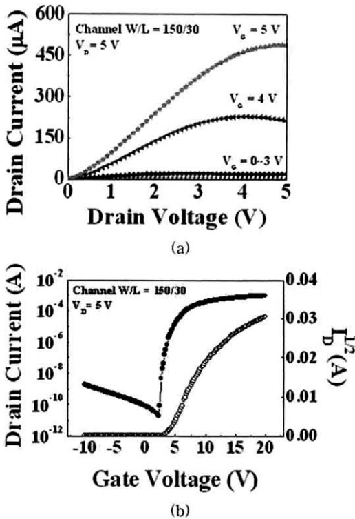
그림 2. 제작된 a-IGZO TFT (channel W/L = 150/30 \mu m )의 전기적 특성 (a) 출력 특성 (b) 전달 특성.
