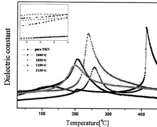
그림 3. 다양한 온도 (1000°C~1150°C)에서 소결한 0.94NKN-0.06BTS 세라믹의 10 kHz에서의 온도변화에 따른 유전상수의 변화. (삽화: 25°C~60°C에서의 확대 이미지)
