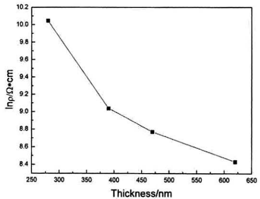
그림 9. 두께 변화에 따른 저항율.
