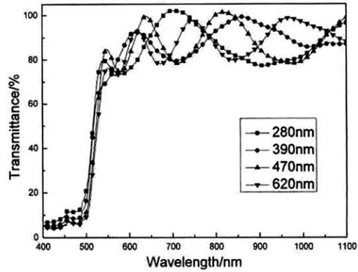
그림 8. 두께 변화에 따른 광 투과율.
