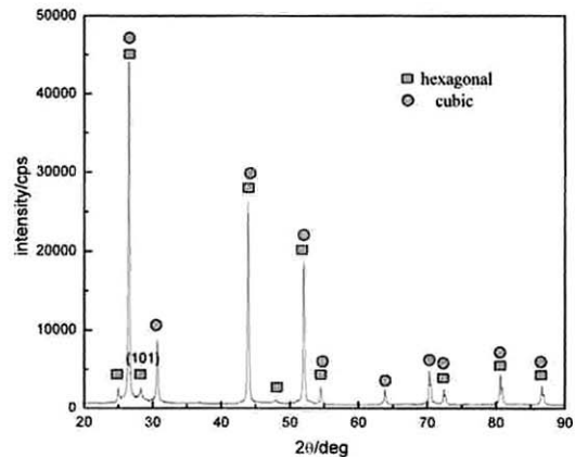
그림 2. CdS 분말의 XRD 패턴. Fig. 2. The XRD patterns of CdS powder.
