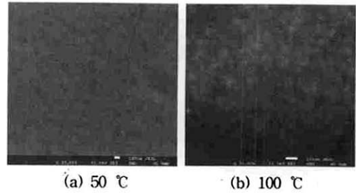
그림 4. 기판온도의 변화에 따른 CdS 박막의 SEM.
