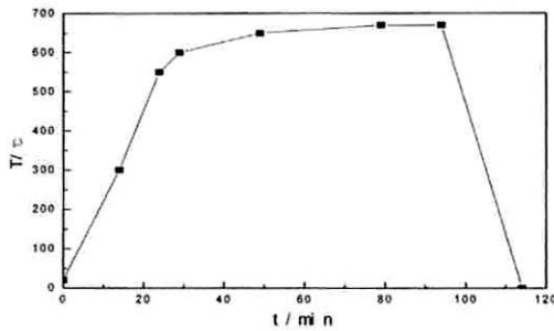
그림 1. CdS분말의 열처리 곡선. Fig. 1. The heat-treatment curve of CdS powder.
