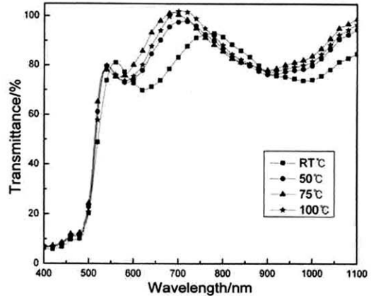
그림 5. 기판온도의 변화에 따른 CdS 박막의 광투과율.
