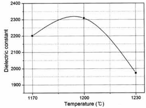
그림 6. BaTiO 3 세라믹의 소결 온도 변화에 따른 비유전율(ε r )의 변화.
