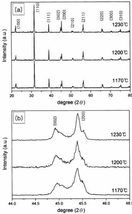
그림 5. 여러 조건으로 제작한 BaTiO 3 소결체의 XRD 회절 도형: (a) 장 범위 측정, (b) 단 범위 측정.
