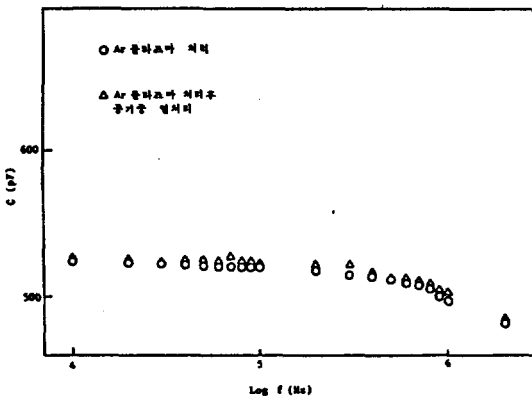
그림 12. 플라즈마 처리한 PPMMA의 주파수-C 특성
