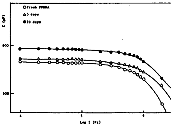
그림 5. 대기중 노출한 PPMMA의 주파수-C특성 Fig 5. Freq vs C of PPMMA exposed to air.
