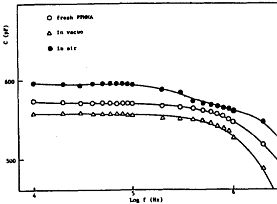
그림 8. 열처리한 PPMMA의 주파수-C 특성 Fig. 8. Freq. vs C of PPMMA treated by annealing.
