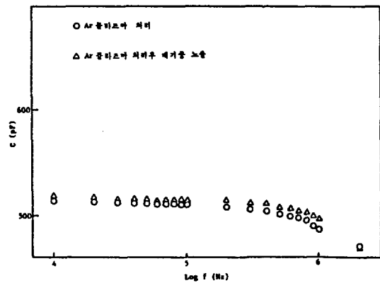
그림 10. 플라즈마 처리한 PPMMA의 주파수-C 특성 Fig. 10. Freq. vs C of PPMMA treated by plasma.
