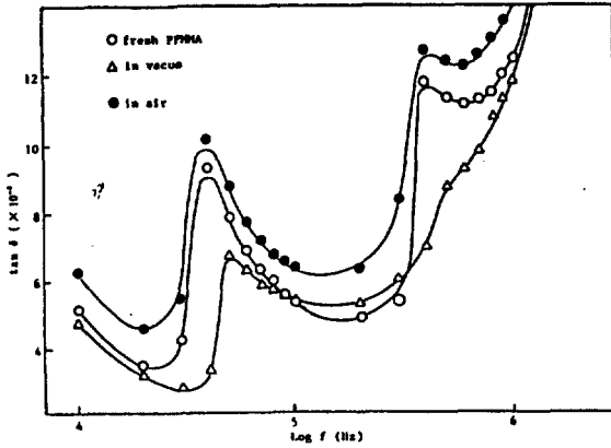
그림 7. 열처리한 PPMMA의 주파수-tan δ 특성 Fig. 7. Freq. vs tan δ of PPMMA treated by annealing.
