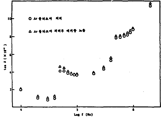
그림 9. 플라즈마 처리한 PPMMA의 주파수-tan δ 특성 Fig. 9. Freq. vs tan δ PPMMA treated by plasma.
