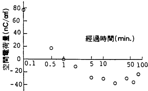
그림 6. 공간전하의 양 Fig.6. The amount of the space charge.
