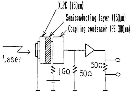
그림 1. 압력파 방법의 원리 Fig.1. Principle of the Pressure pulse method.
