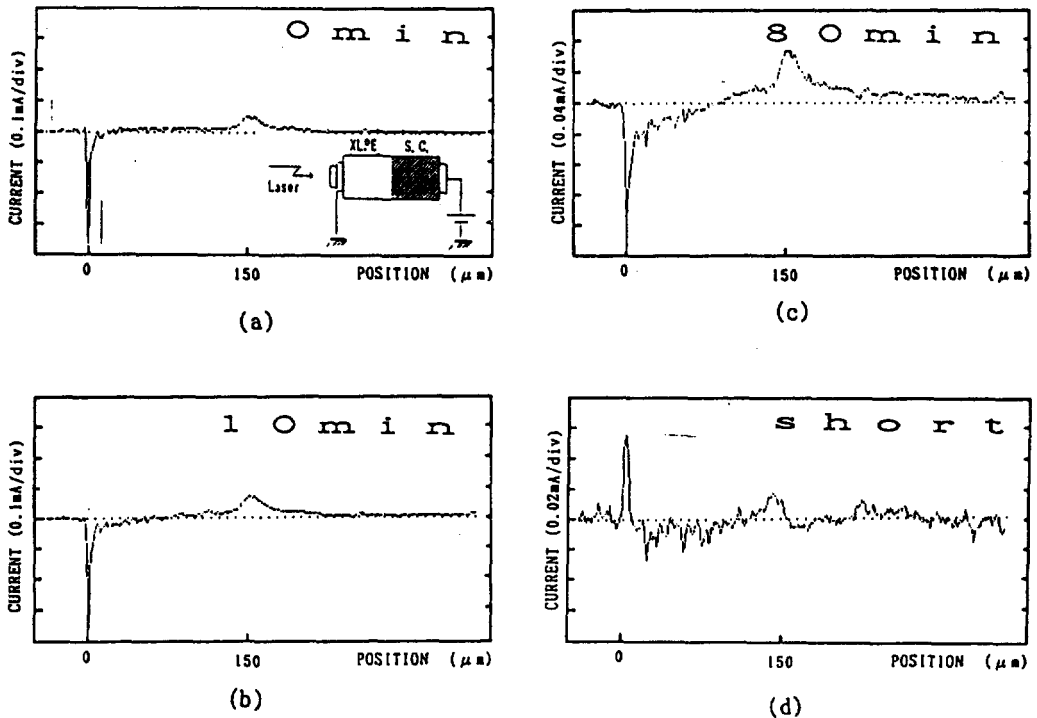
그림 5. 양극이 반도체층인 XLPE에서 LIPP 특성
