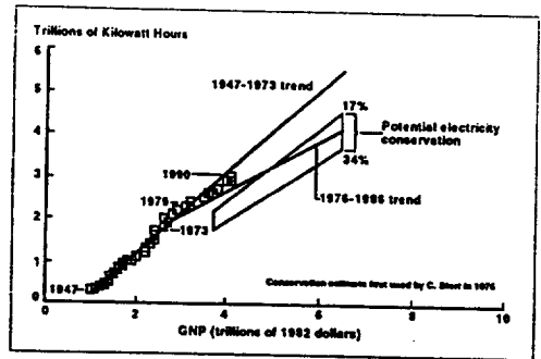
그림 2 미국내에서 GNP대 전기에너지 소비량의 절감효과
