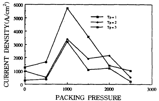
그림 5. 초기충진압력에 따른 초전도데이터의 임계전류밀도(Tp : 테이프화를 위한 가압횟수)
