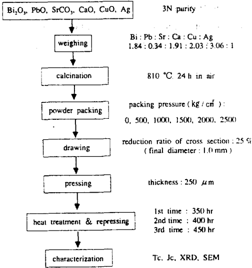
그림 1. 시편 제작 공정도
