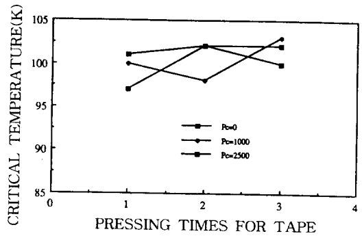
그림 7. 테이프화를 위한 가압횟수에 따른 초전도테이프의 임계온도(Pc : 초기충진압력)
