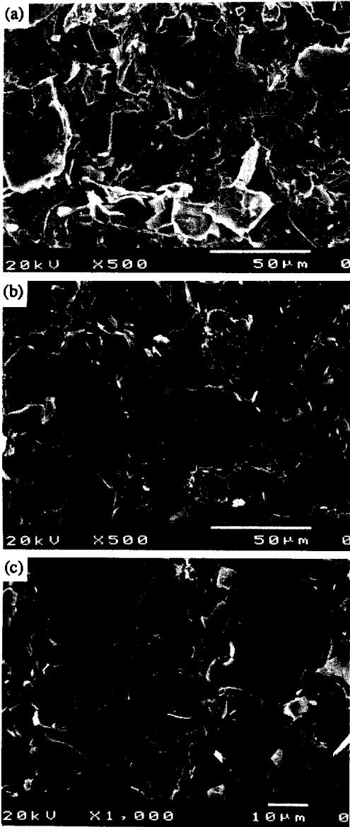
사진 2. 테이프화를 위한 가압횟수에 따른 초전도 테이프의 주사전자현미경 사진(초기충진압력 : 1000\text{kg/cm}^2 ) (a) 1회 (b) 2회 (c) 3회
