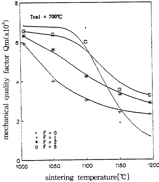
그림 7 소결온도에 따른 기계적품질계수 Fig. 7 Mechanical quality factor vs. sintering temperature for flux contents.
