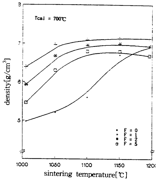
그림 4 소결온도에 따른 시편의 소결밀도 Fig. 4 Fired density vs. sintering temperature for samples calcined at 700°C
