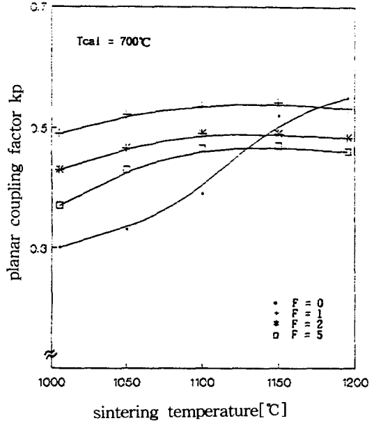
그림 6 소결온도에 따른 시편의 경방향 전기기계결합계수 Fig. 6 Planar coupling factor vs. sintering temperature for flux contents
