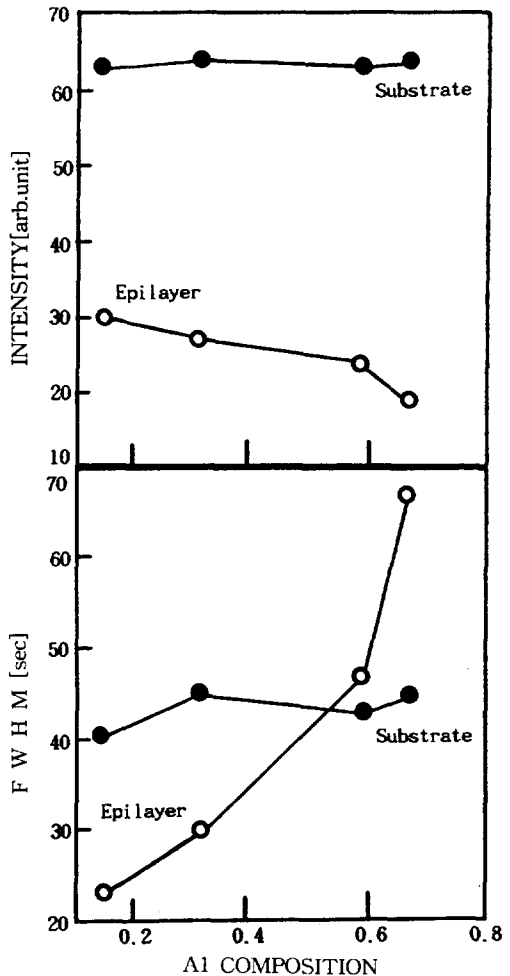
그림 6 조성비에 대한 GaAs 기판과 Al x Ga 1-x As 에피층에서 강도와 반치폭 변화.
