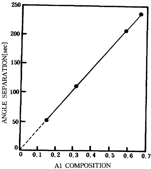
그림 5 Al x Ga 1-x As 에피층에서 조성비에 따른 각도 분리의 변화.
