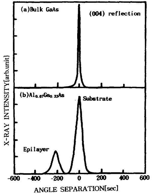
그림 3 (a) bulk GaAs와 (b) Al_{0.67}Ga_{0.33}As 에피층의 (004) 반사면에 대한 이중결정 X-선 회절모양
