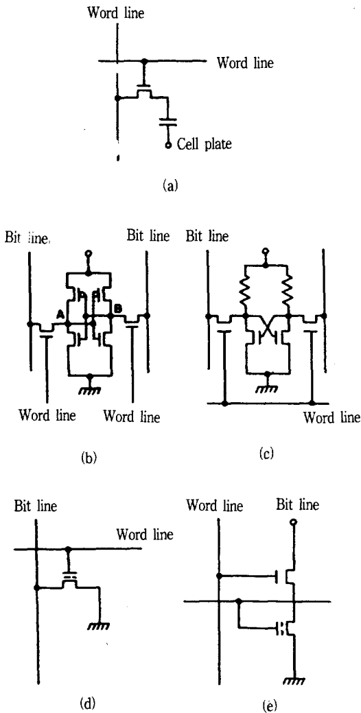
그림 2 기본적인 반도체 메모리 셀
