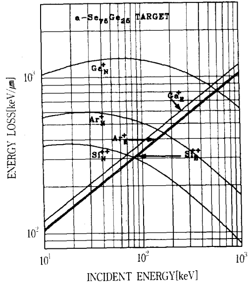
그림 1. Si ++ , Ar ++ , Ga ++ 이온에 대한 비정질 Se 75 Ge 25 레지스트의 에너지손실(dE/dx) N,E
