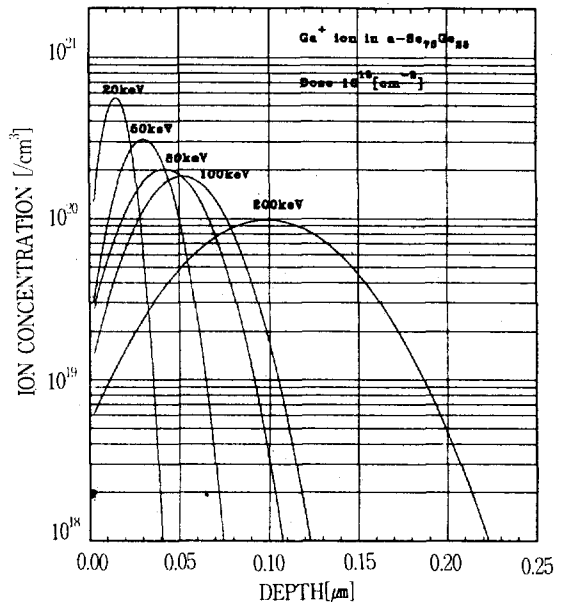
그림 4. 에너지 변화에 따른 비정질 Se 75 Ge 25 레지스트내로 주입된 Ga + 이온 농도 분포
