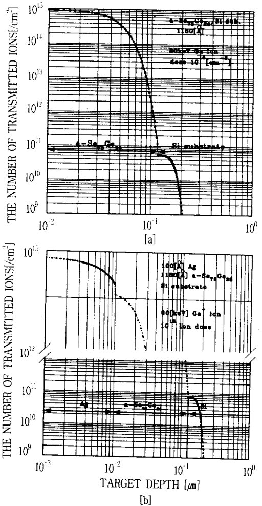
그림 6. 80[keV] 입사에너지, 1×10 15 [cm -2 ] dose의 Ga + 이온에 대한 투과이온수 변화 (a) 0.118[μm] a- Se_{75}Ge_{25} /Si 기판 구조 (b) 0.01[μm] Ag/0.118[μm] a- Se_{75}Ge_{25} /Si 기판 구조
