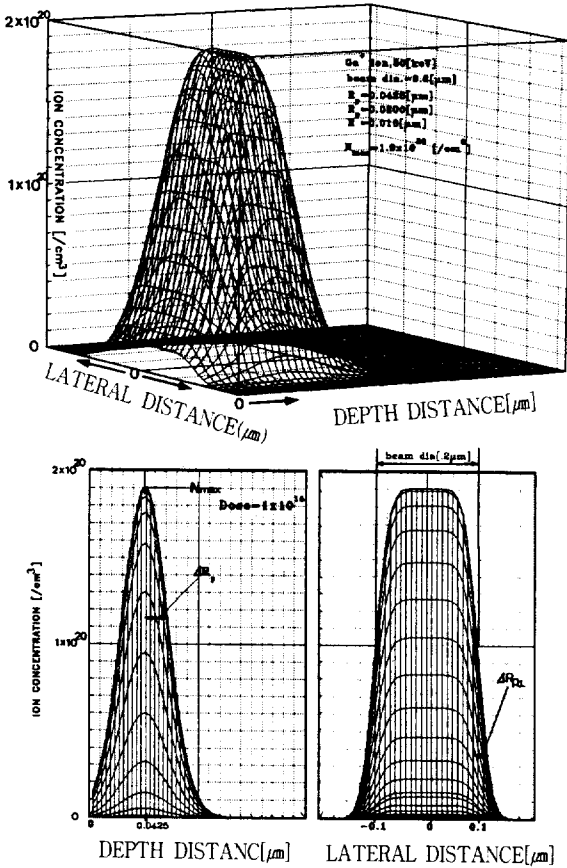
그림 5. 80[keV] 입사에너지, 0.1[μm] 유효빔 반경 및 1×10 15 [cm -2 ] dose의 Ga + 이온에 대한 비정질 Se_{75}Ge_{25} 레지스트 내로 주입된 3차원 농도 분포
