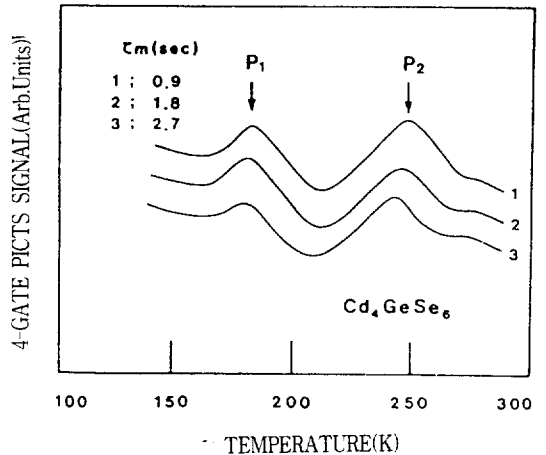
그림 6. Cd 4 GeSe 6 단결정의 4-gate PICTS 신호 Fig. 6. 4-gate PICTS signal of Cd 4 GeSe 6 single crystals.
