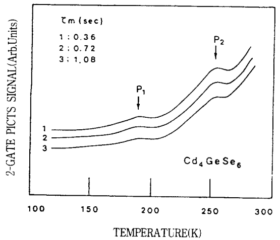
그림 5. Cd 4 GeSe 6 단결정의 2-gate PICTS 신호 Fig. 5. 2-gate PICTS signal of Cd 4 GeSe 6 single crystals.
