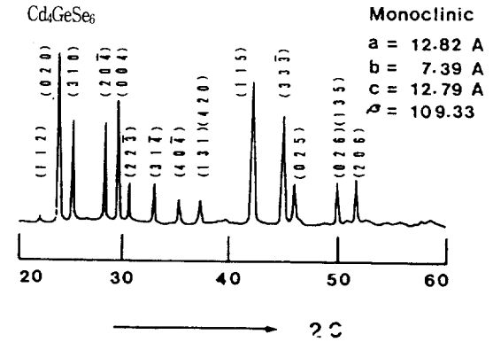
그림 2. Cd 4 GeSe 6 단결정의 X-선 회절무늬 Fig. 2. X-ray diffraction patterns of Cd 4 GeSe 6 crystalline powder.
