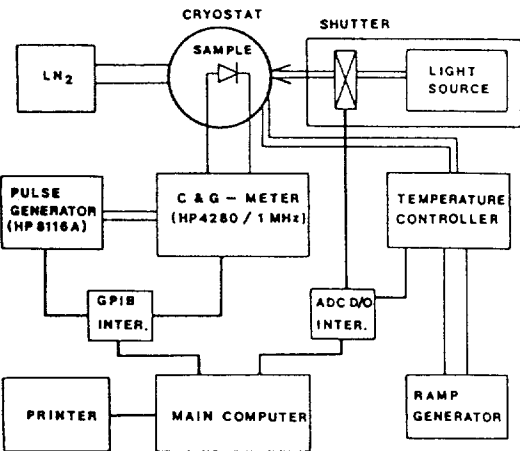
그림 4. PICTS 측정장치의 개략도 Fig. 4. Block diagram of PICTS measurement system.
