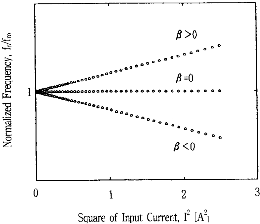
그림 3. 입력전류의 제곱에 대한 규격화 시킨 공진주파수
