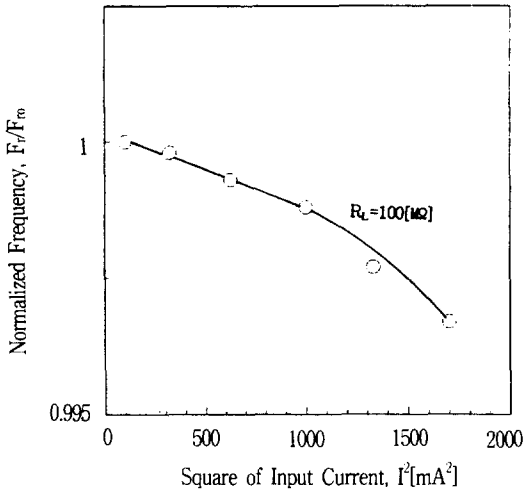
그림 11. 공진전류의 제곱에 대한 규격화시킨 공진주파수. ( R_L=100[M\Omega] ).
