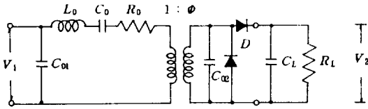
그림 1. 압전변압기의 등가회로 Fig. 1. Equivalent circuit of the piezoelectric transformer.
