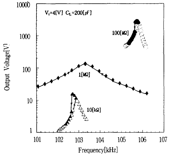
그림 13. 부하저항에 대한 출력전압의 공진특성 ( V_i=4V ).
