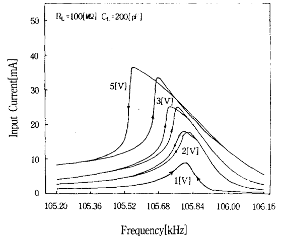
그림 10. 입력전류의 공진특성( R_L=100[m\Omega] ).
