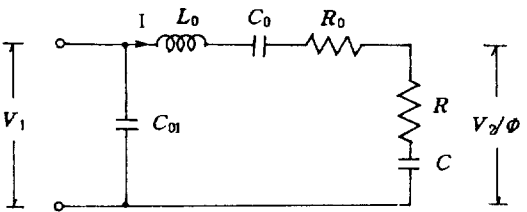
그림 2. 1차측에 환산한 등가회로 Fig. 2. Equivalent circuit converted to the primary-side.
