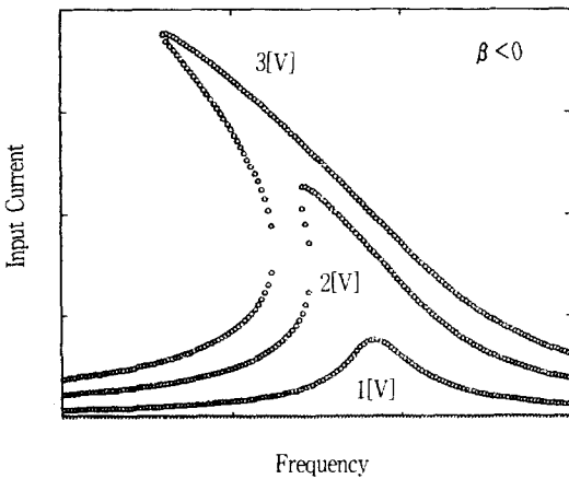
그림 6. 입력전압에 대한 입력전류의 공진특성 ( \beta < 0 ). Fig. 6. Resonance characteristics of input current as a function of input voltage ( \beta < 0 ).
