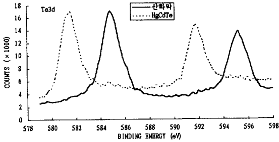
그림 10. 텔루륨의 화학적 상태 Fig. 10. Chemical state of Te.
