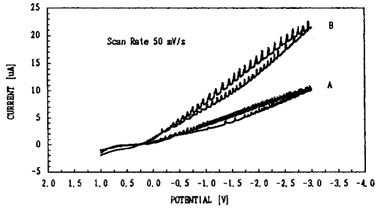
그림 5. H 2 O 2 용액에서의 순환 전류-전압 관계 Fig. 5. Cyclic Voltammery in H 2 O 2 .
