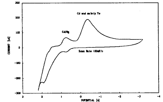
그림 6. KOH 용액에서의 순환 전류-전압 관계 Fig. 6. Cyclic Voltammery in KOH.
