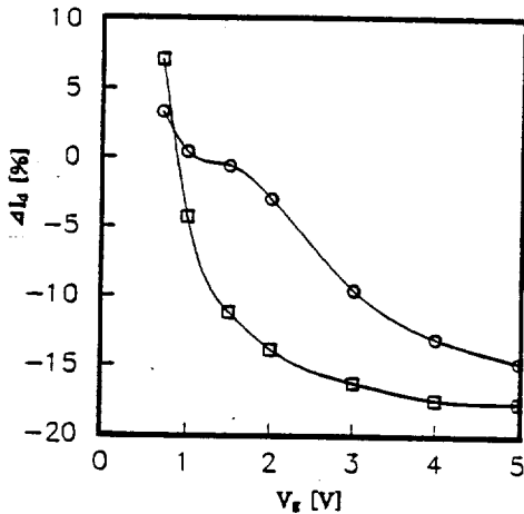
그림 3. 게이트 전압에 따른 드레인 전류의 변화
