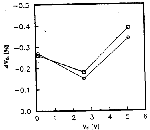
그림 2. 드레인 전압에 따른 문턱 전압의 변화 V_b = -2 Fig. 2. The variation of the threshold voltage due to the drain voltage V_b = -2V
