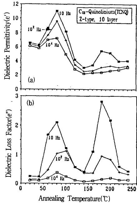
그림 7. 10, 10^2 , 10^4 Hz에서의 열처리 온도에 따른 C_{22} -Quinolinium(TCNQ) LB막의 (a) 실수부 유전율과 (b) 허수부 유전율.
