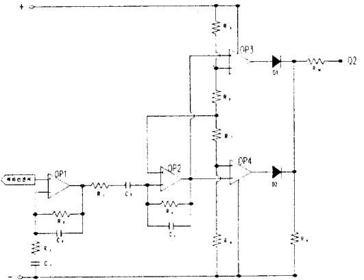
그림 3. 적외선 센서 신호 증폭단 Fig. 3. Circuit of amplifier for IR sensor signal.
