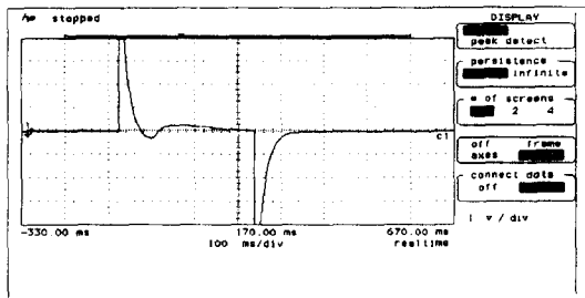
그림 6. 적외선 센서신호 증폭부의 출력파형 Fig. 6. Output signal of amplifier for IR sensor signal.
