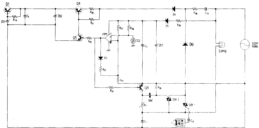
그림 1. 회로동작용 전원공급부, 광도전센서 증폭부 및 조광부
