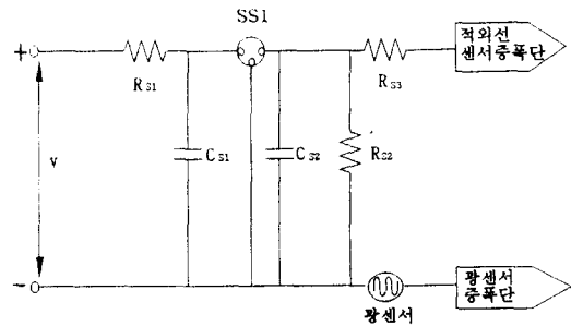
그림 2. 센서단 회로
