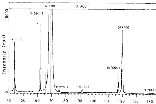
그림 4. 다이아몬드막(그림 2-a)의 X-선 회절도
