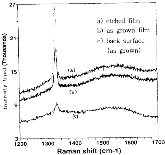
그림 5. 다이아몬드막(그림 2)의 Raman스펙트럼 Fig. 5. Raman spectrum of the diamond films shown in fig. 2.
