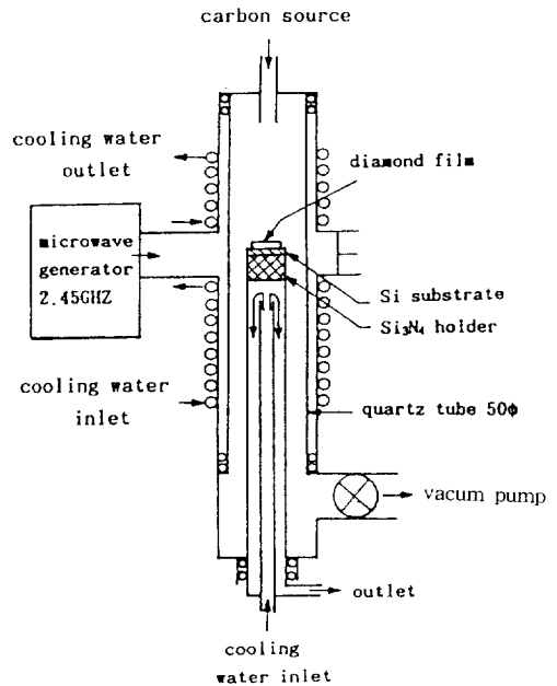
그림 1. 실험장치의 개략도
