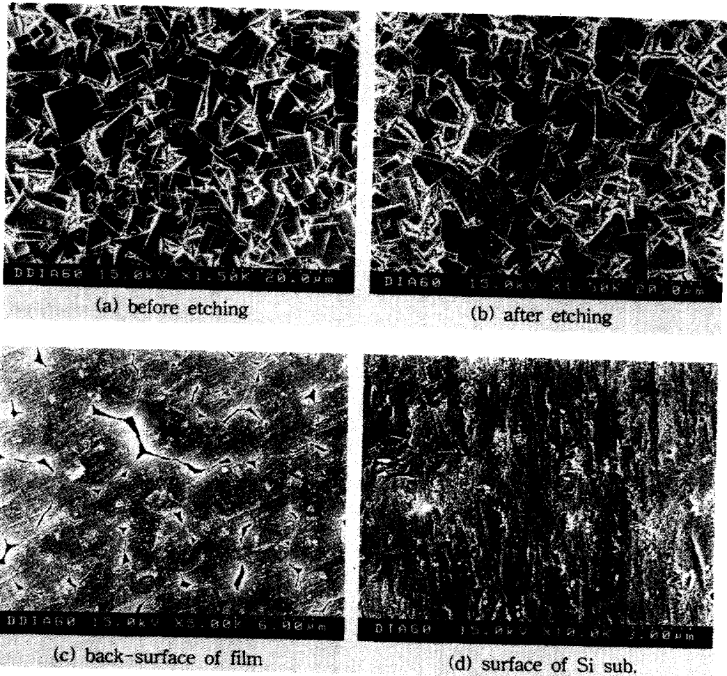
그림 2. 메탄농도 3%로 실리콘기판 위에 20시간 성장시킨 다이아몬드막의 SEM사진 Fig. 2. SEM photographs of the diamond films deposited for 20 hours on silicon substrate at CH_4/H_2 = 3\% .
