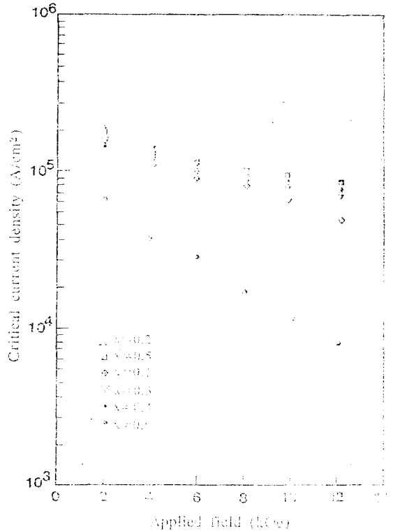
그림 3. 30K 온도에서 Y_{1-x}Yb_xBa_2Cu_3F_xO_7 계의 임계전류밀도에 대한 자기장 의존성
