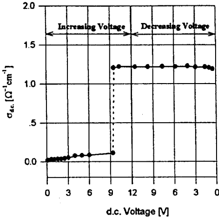
그림 2. d.c.바이어스에 의한 d.c.전도도의 특성 곡선(두께:1 \mu m, 열처리 온도:393K, 열처리 시간:2 hours, 전극간 간격:3mm) Fig. 2. d.c. conductivity characteristic curve with d.c. bias(thickness:1 \mu m, annealing temperature:393K, annealing time:2 hours, and separation between d.c. electrodes:3mm).
