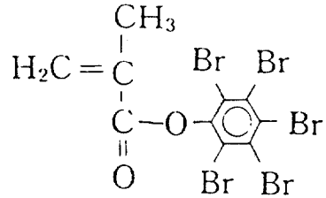
그림 3. Pentabromovinylmetaglrade의 화학구조
